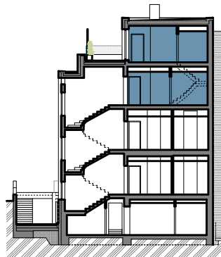
SCHÉMATICKÝ ŘEZ
