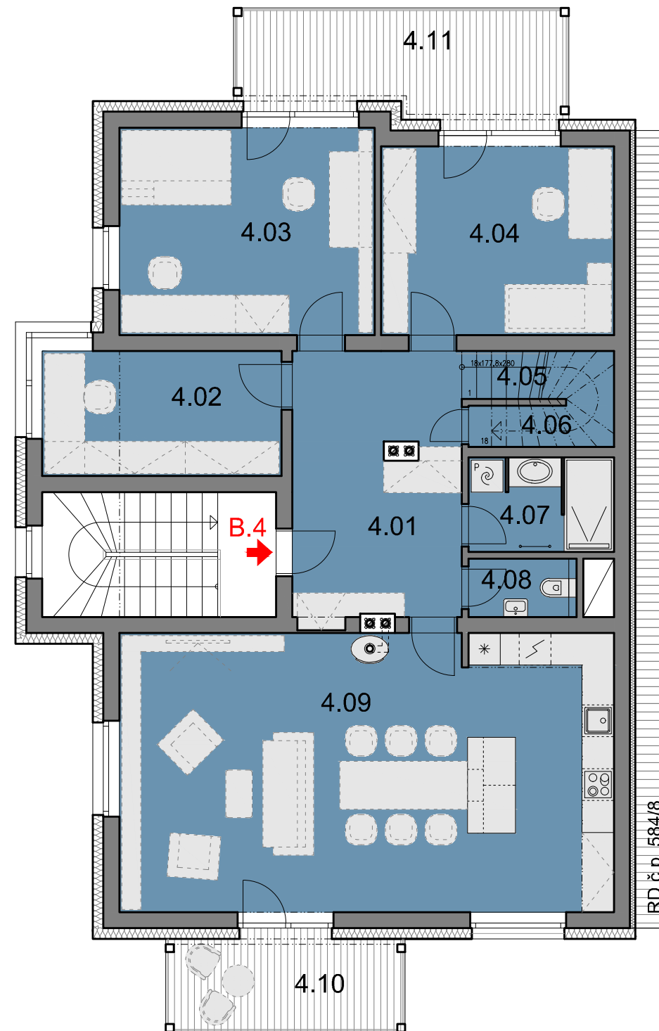
4.NP – PŮDORYS 1:100
