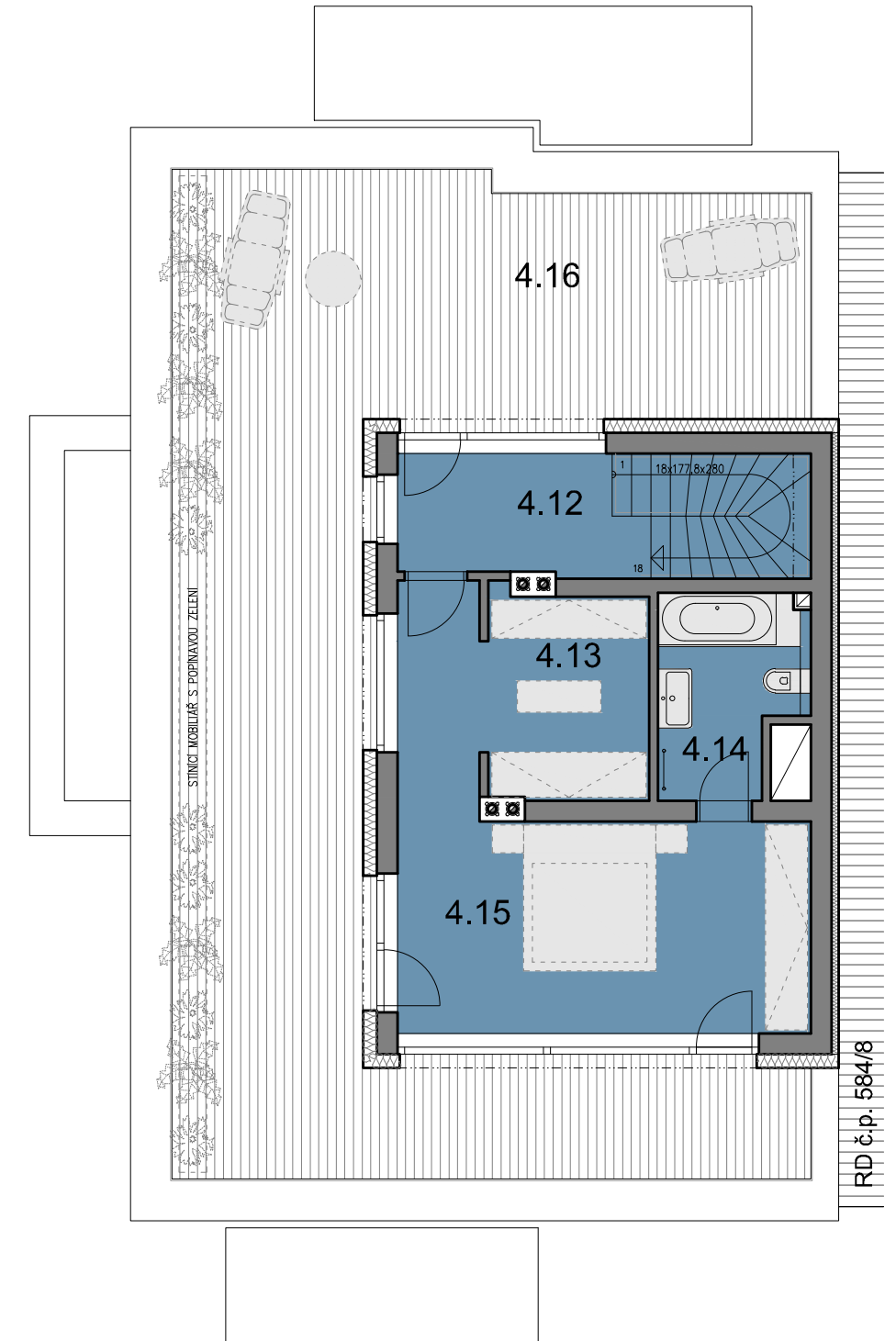
5.NP – PŮDORYS 1:100
